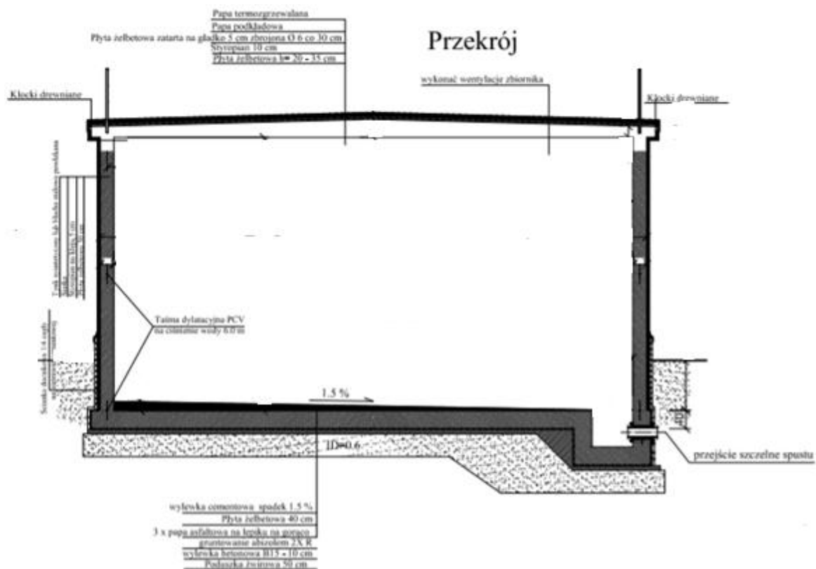
Rys. 2 – przekrój zbiornika
