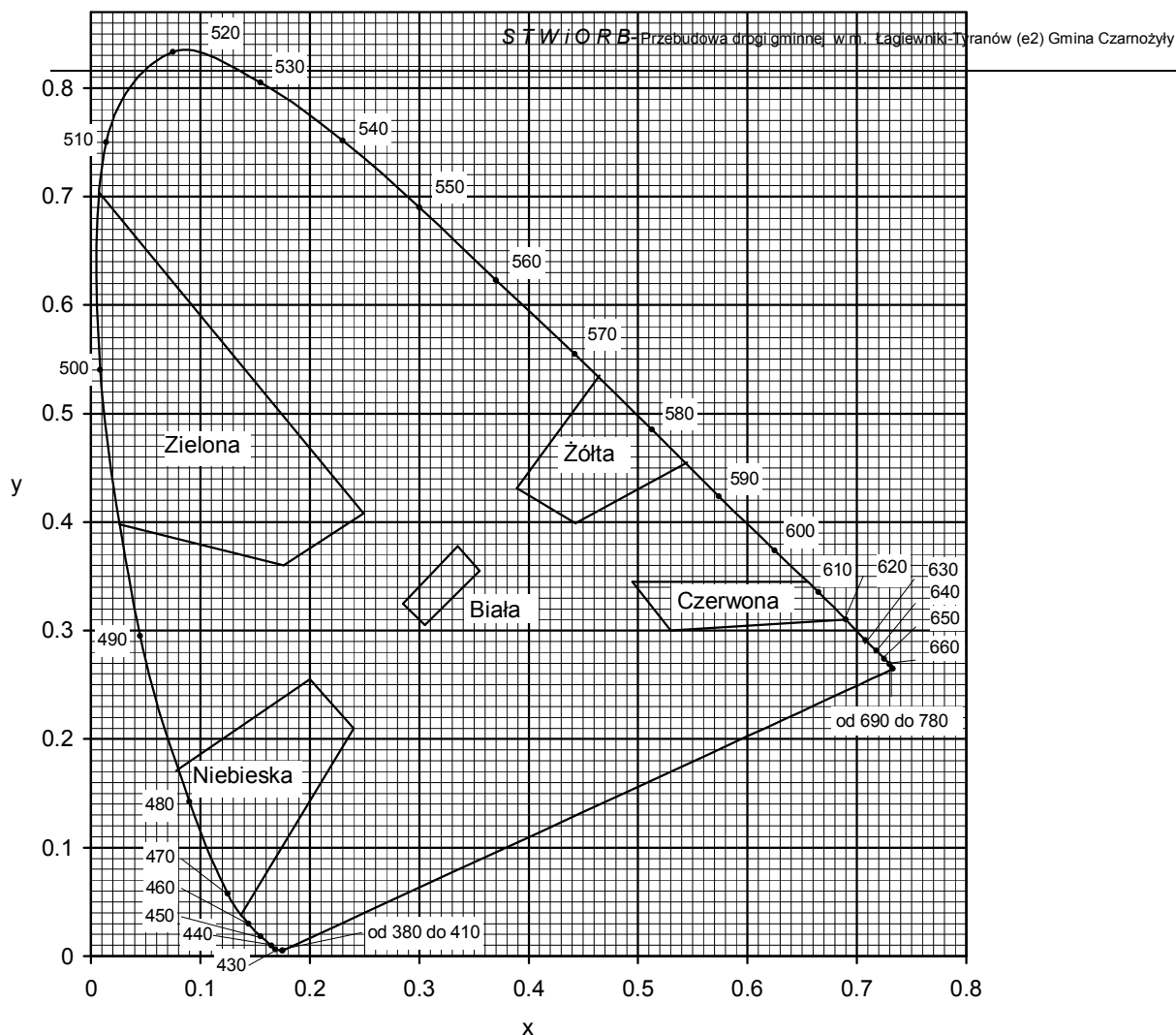
Rys. 2. Granice barw białej, żółtej, czerwonej, niebieskiej i zielonej oznakowania
